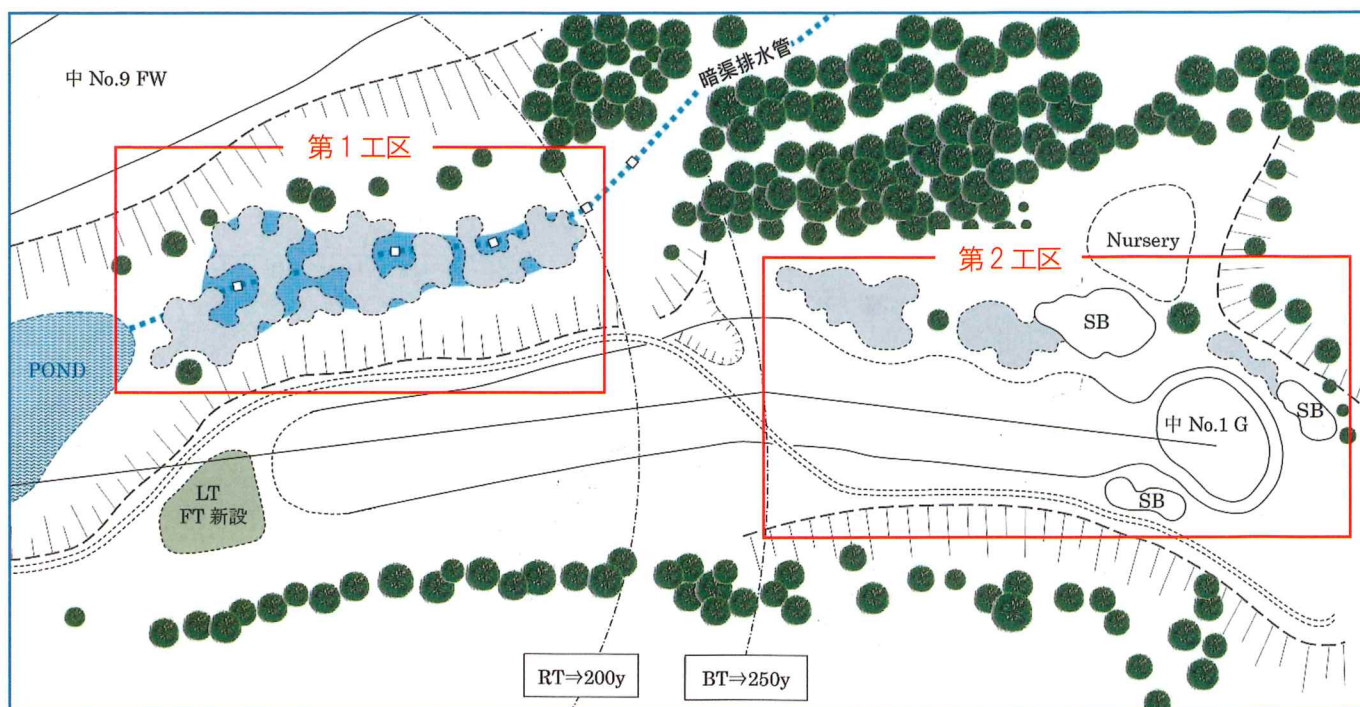
■中 No.1 バンカー改修工事図
